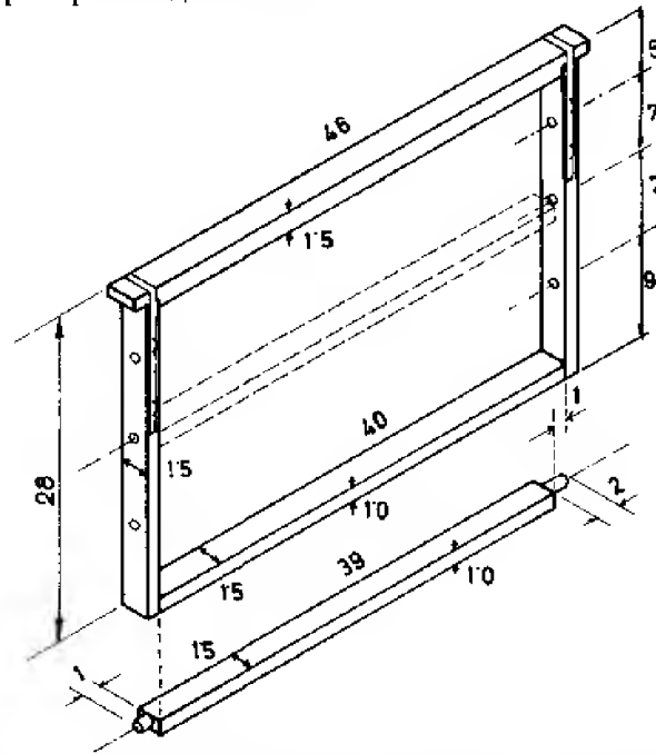
Специјални оквир са 3 покретне лајснице на које се лепе вештачке матичне основце при производњи матица или млеча (мере изражене у мм)
